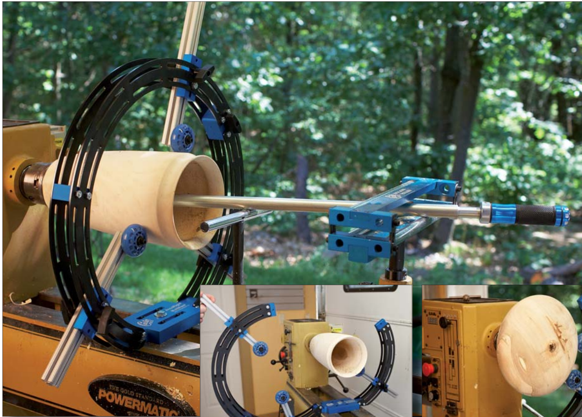
Люнет MultiRest Артикул: SR1000
